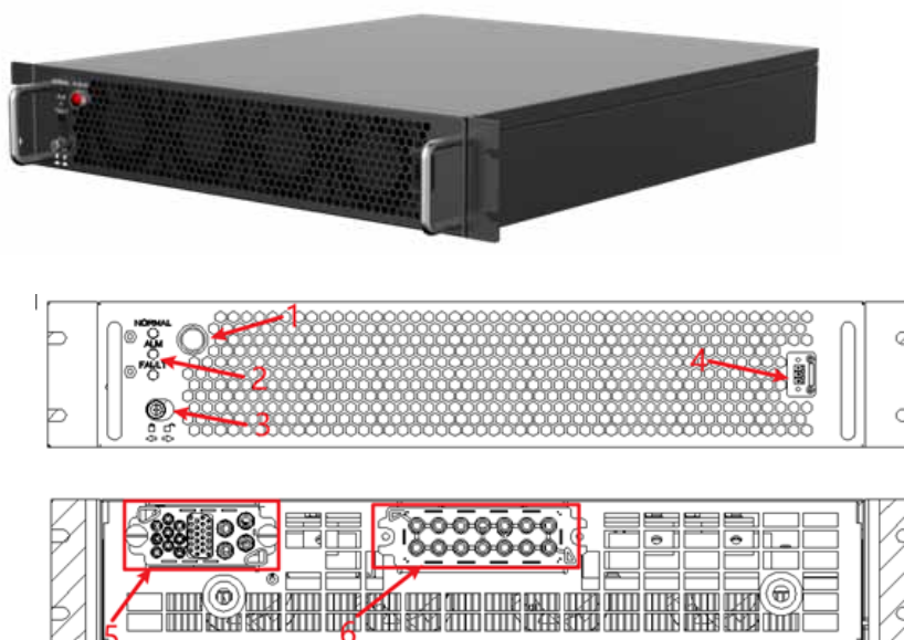
Рисунок 3-4 Модуль байпаса
